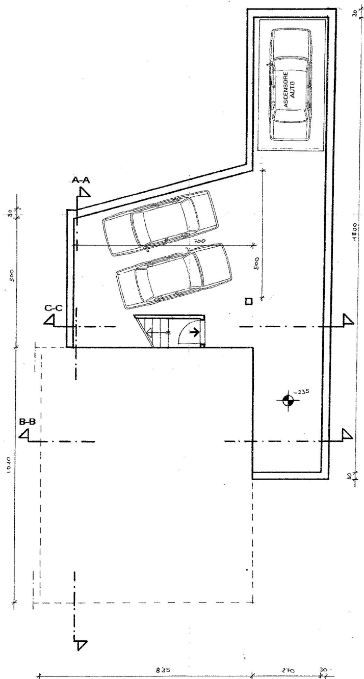
PIANO SOTTERRANEO
